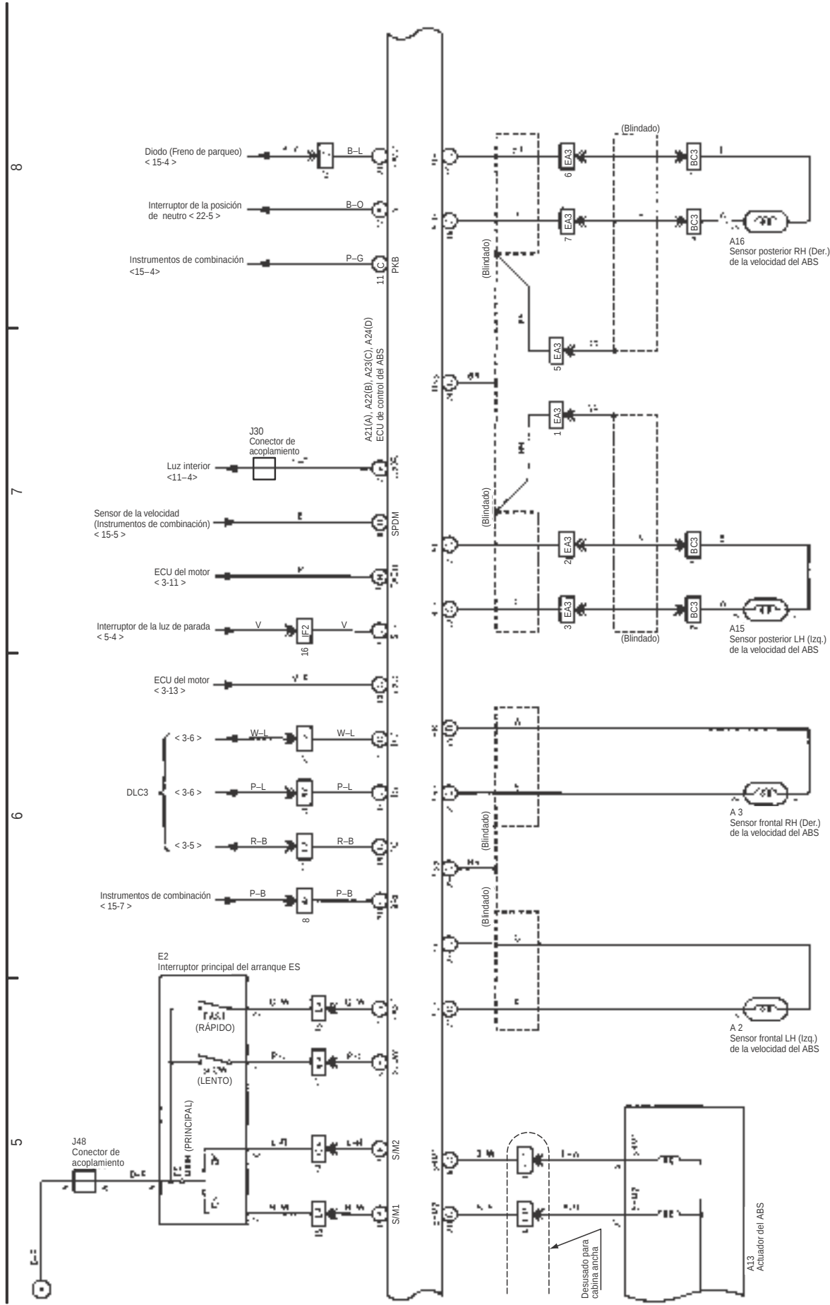
Sistema del ABS y del arranque ES (N04C-TF)
